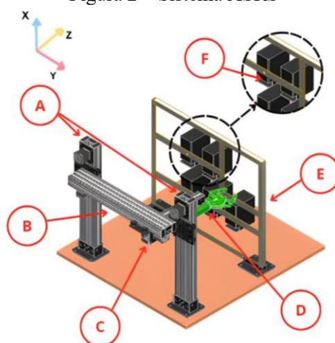
Figura 2 – Sistema ASRS
